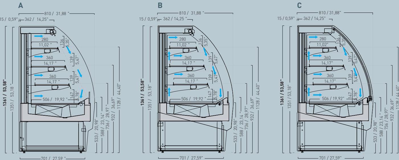
ALTEZZA PIANI ESPOSITIVI VARIABILE TRAMITE CREMAGLIERA Height of display shelves adjustable by rack / Hauteur étagères d'exposition réglable par crémaillère Höhe der Ausstellflächen mittels Zahnschiene einstellbar / Altura de los tableros de exposición variable mediante cremallera
